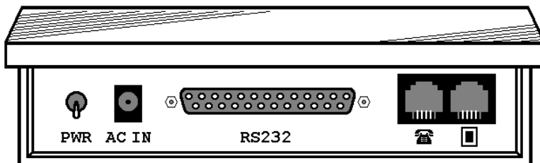
Рис. 1. Задняя панель модема
